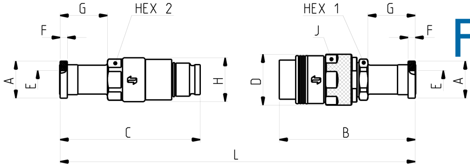
Flange Head Adapter - Codolo per Flangia - Flanschtelleradapter - Fixation raccordement Bride (ISO 6162-2)
