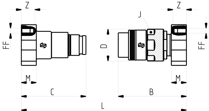
Flange Adapter - Adattatore con Flangia - Flanschadapter - Reccordement Bride (ISO 6162-2)
